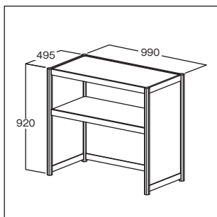
受付カウンター(中棚付き) W990 D495 H920
