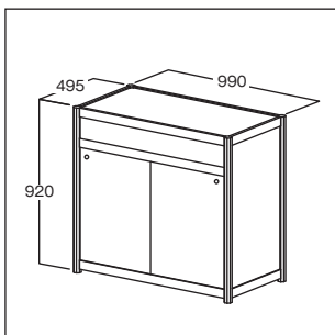
展示台(引き戸付) W990 D495 H920
