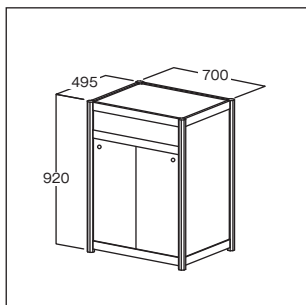
展示台(引き戸付) W700 D495 H920
