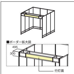
行灯ボーダー W2,970 D495 H300
