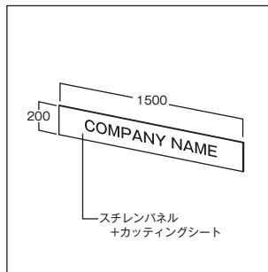
ロゴサインボード(データ支給) W1,500 H200
