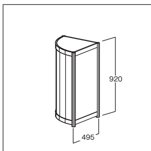
R型展示台 W495 D495 H920
