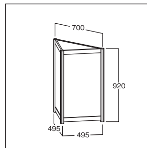
三角展示台 W700 D495 H920
