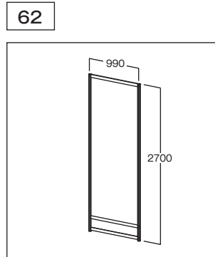
壁面パネル W990 H2,700
