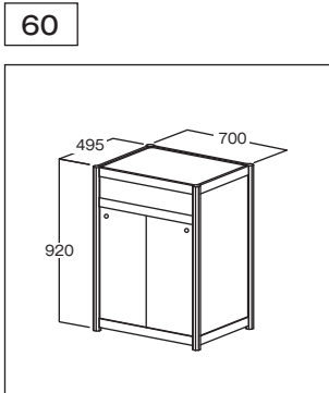
展示台(引き戸付) W700 D495 H920
