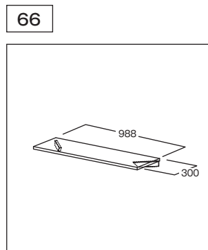
棚ユニット W988 D300
