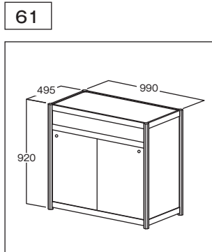
展示台(引き戸付) W990 D495 H920
