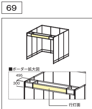
行灯ボーダー W2,970 D495 H300
