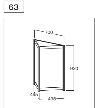
三角展示台 W700 D495 H920
