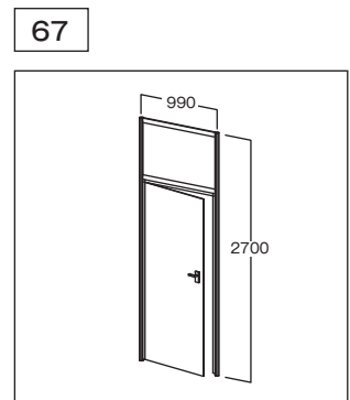
ドアパネル(鍵付き) W990 H2,700
