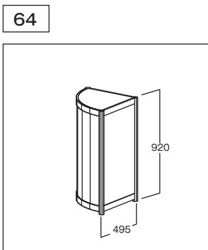
R型展示台 W495 D495 H920
