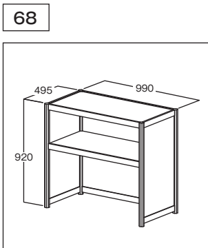
受付カウンター(中棚付き) W990 D495 H920
