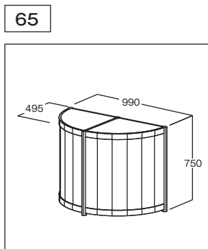
R型展示台 W990 D495 H750
