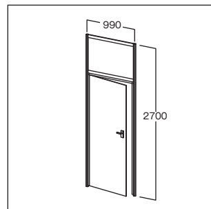
ドアパネル(鍵付き) W990 H2,700
