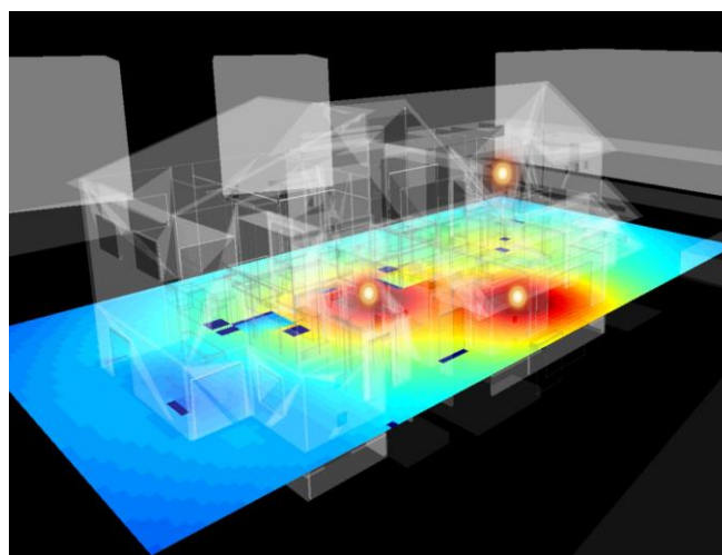
図 2 実験住宅 2 棟での大規模電磁界解析例
