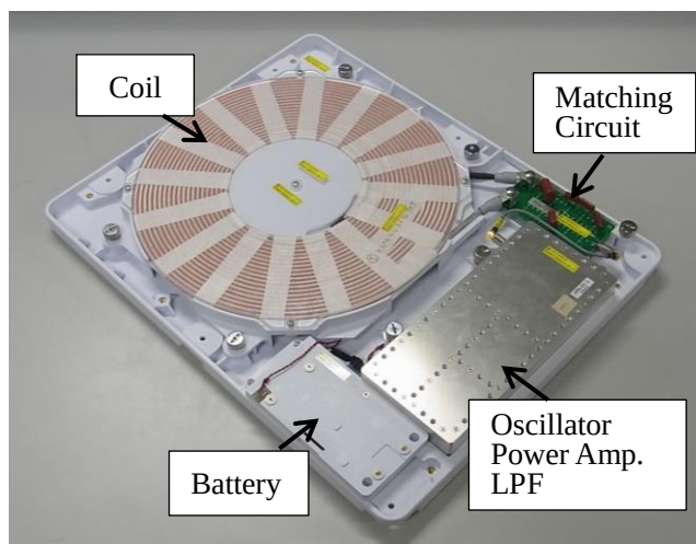
図 1 WPT エミュレータの内部構成
