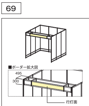
行灯ボーダー W2,970 D495 H300
