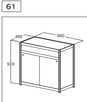
展示台(引き戸付) W990 D495 H920
