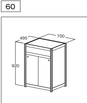
展示台(引き戸付) W700 D495 H920
