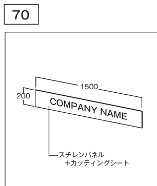
ロゴサインボード(データ支給) W1,500 H200
