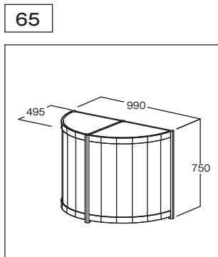
R型展示台 W990 D495 H750
